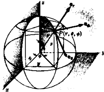
Fig. 22-13. Coordenadas esféricas.
